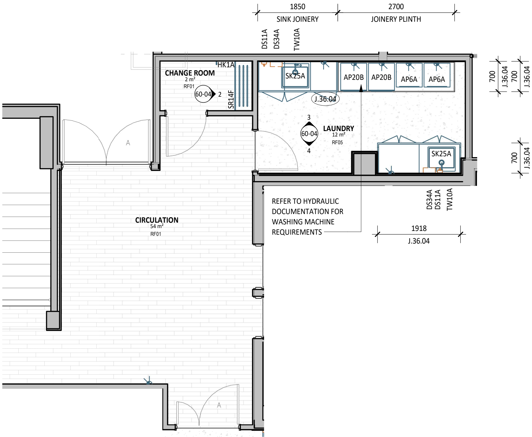
1 PLAN DETAIL 1 : 50
