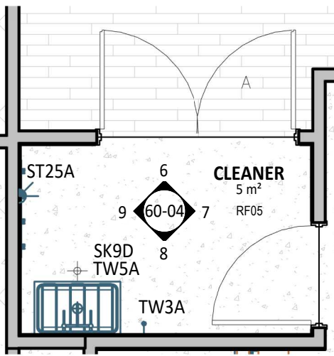
5 PLAN DETAIL 1 : 50
